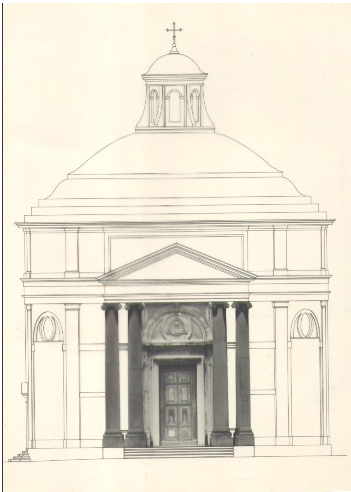
Restituzione della facciata principale - originale in scala 1.50.
