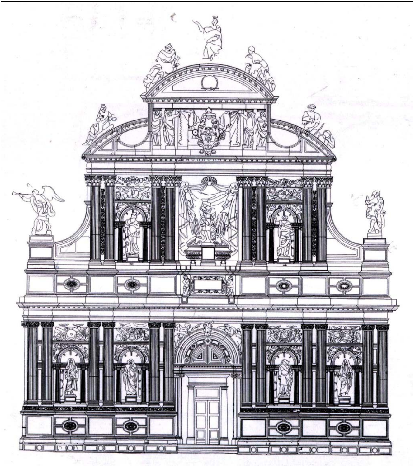
Restituzione fotogrammetrica al tratto della facciata principale - originale in scala 1:20.
